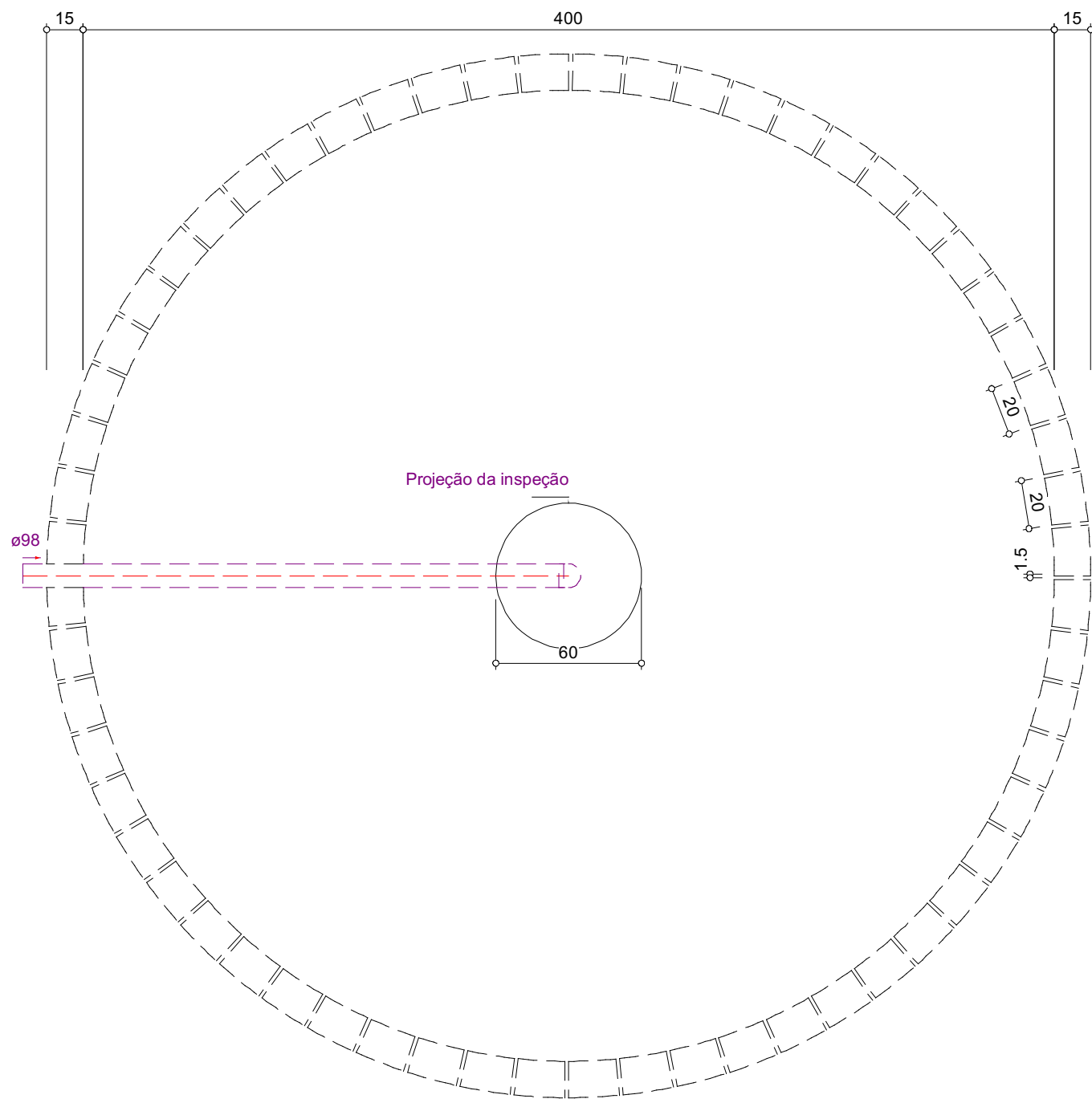
Sumidouro - TÉRREO Planta baixa - ESC. 1:25
