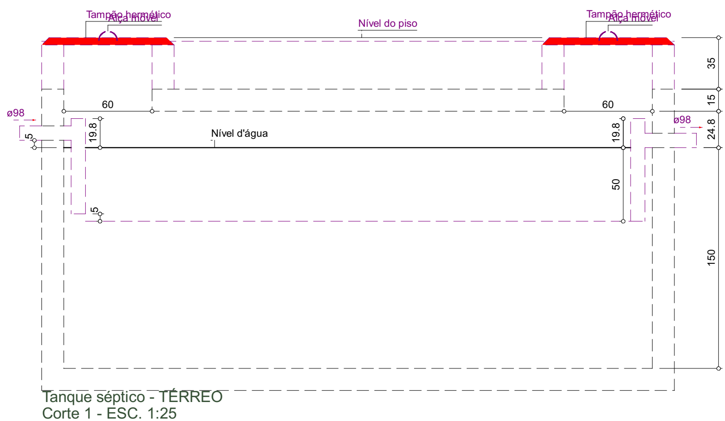
Tanque séptico - TÉRREO Corte 1 - ESC. 1:25
