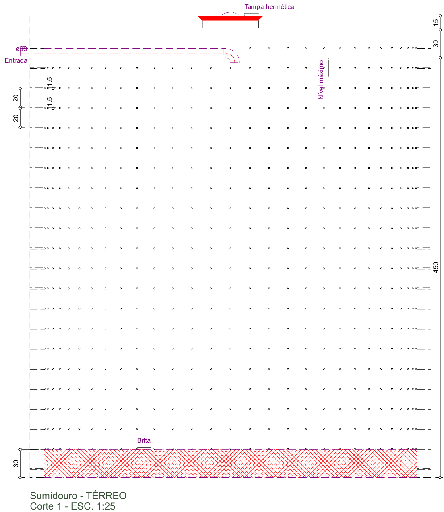
Sumidouro - TÉRREO Corte 1 - ESC. 1:25
