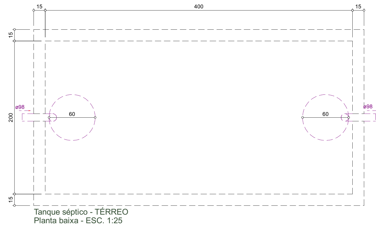
Tanque séptico - TÉRREO Planta baixa - ESC. 1:25
